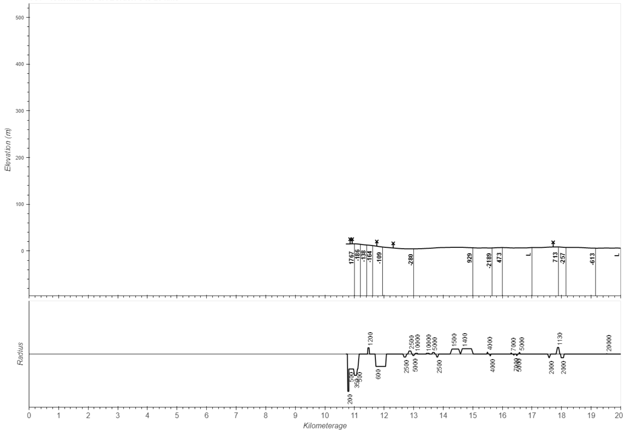
V01 - Tottenham to SA Border: 0 to 20 kms
